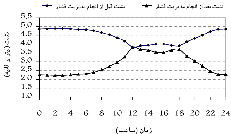
شکل ۵- مقدار نشت ساعتی در شبکه
