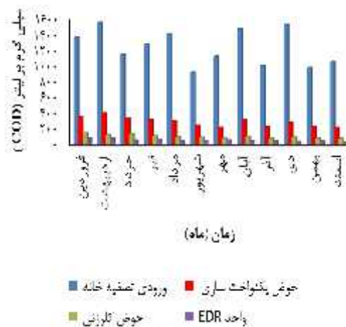
نمودار ۲- مقایسه کارایی واحدها در حذف COD
